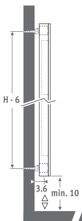
standaard beugels
