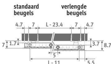
verlengde beugels
