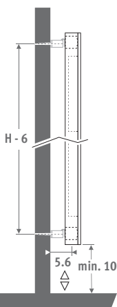
verlengde beugels
